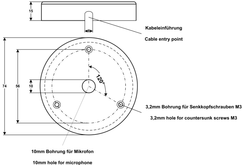
Skizze Montageflansch (Artikelnummer 77200002)
